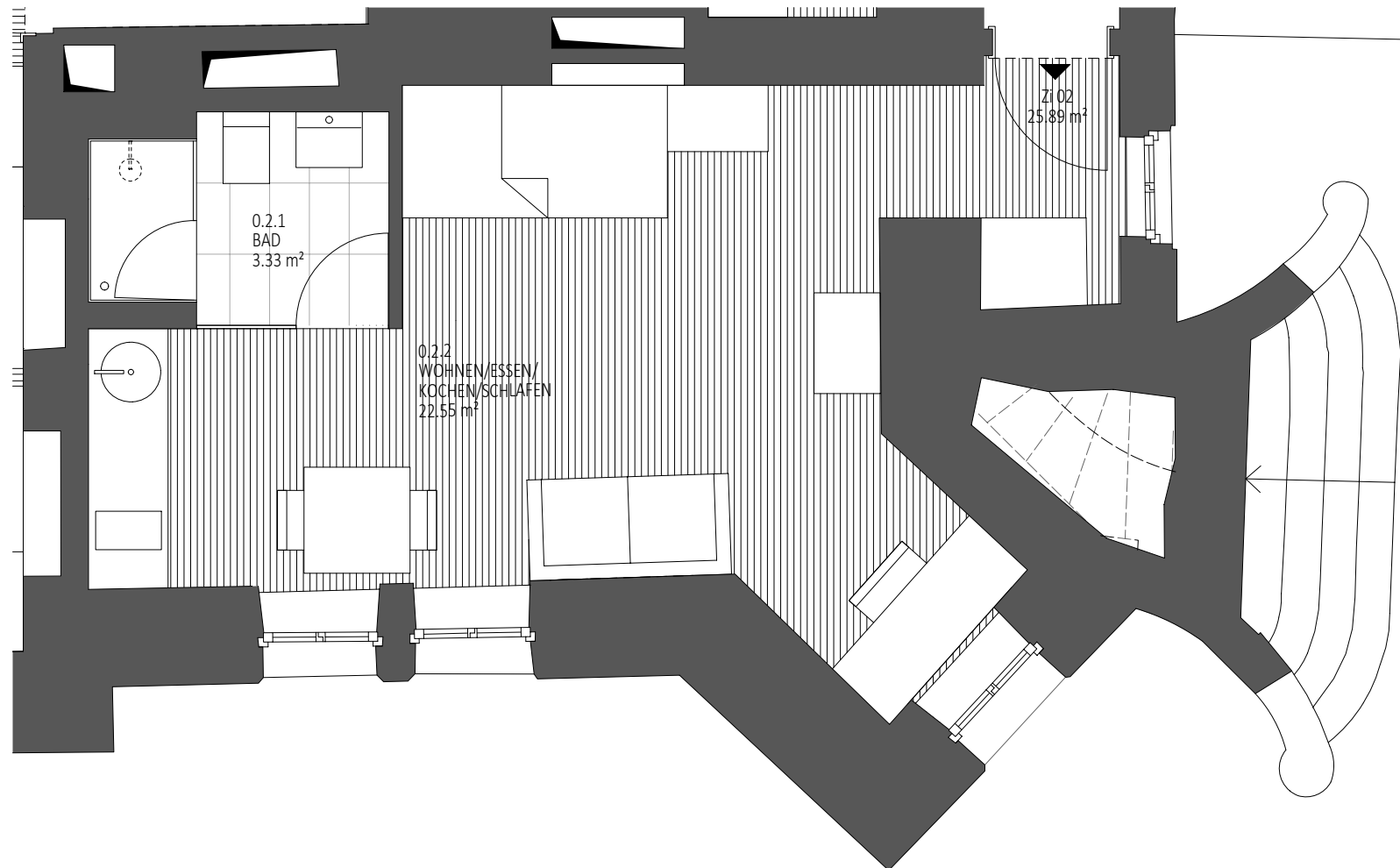
Grundriss UG_WE 2
