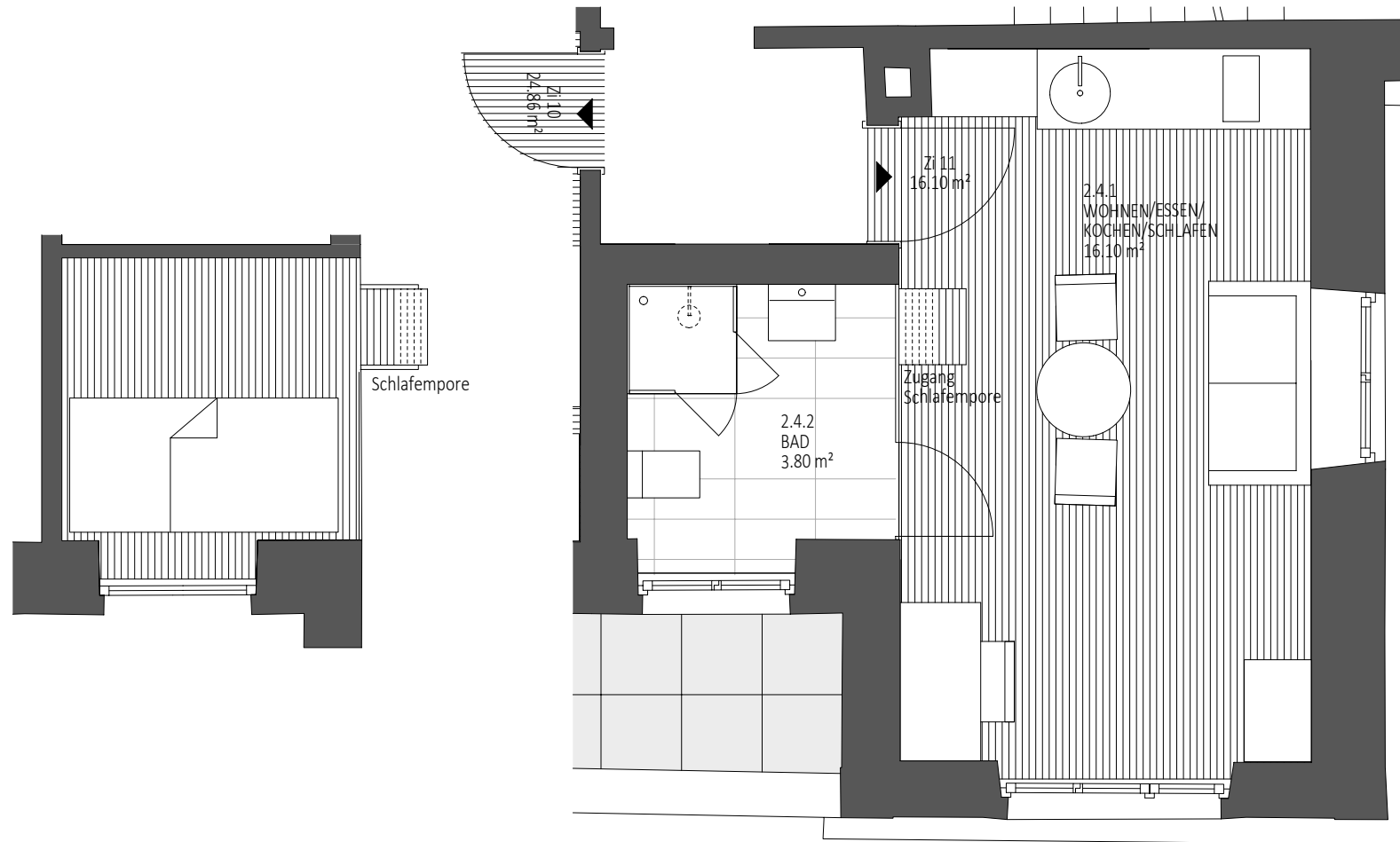
Grundriss 1.OG_WE 11
